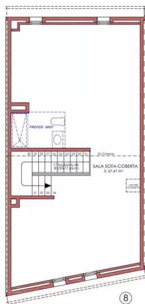
PLANTA GOLFES-COBERTA
