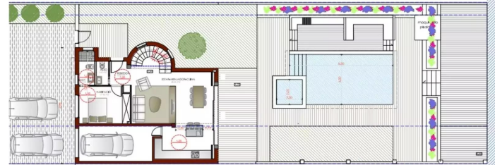
PROPOSTA-P.BAICA-1,100
